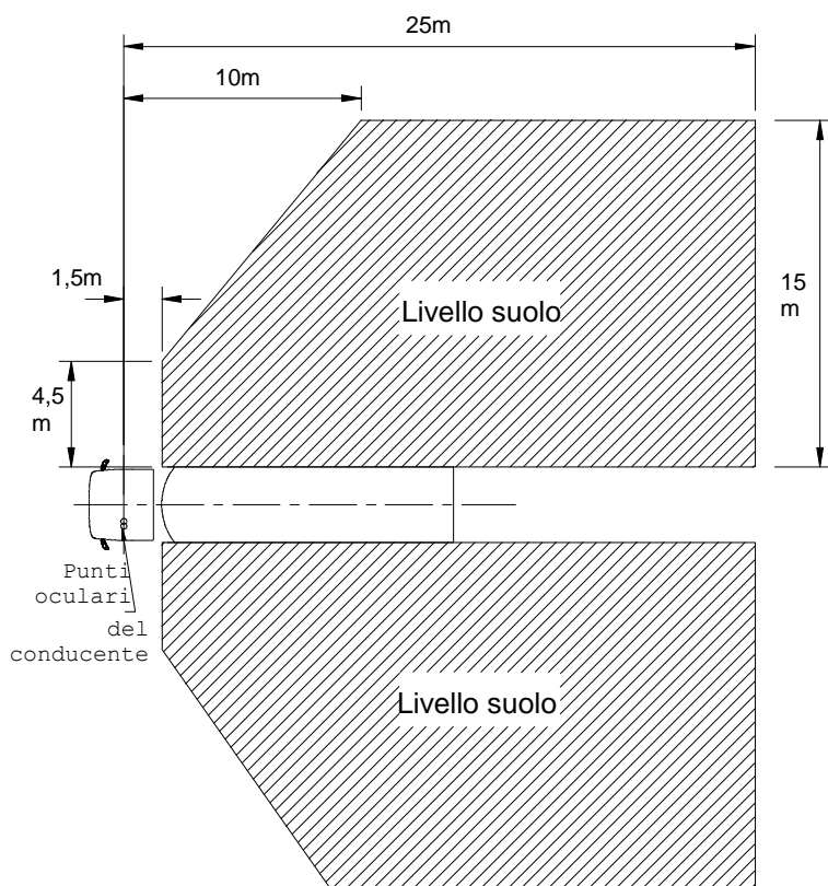
Figura 9: campo di visibilità degli specchi grandangolari della categoria IV
